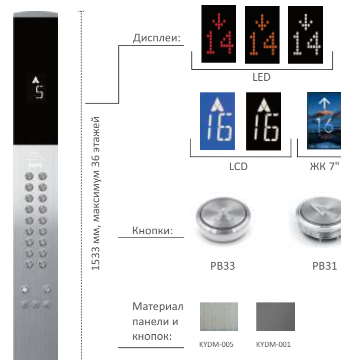
CEC300 (монтируется вровень с поверхностью)
