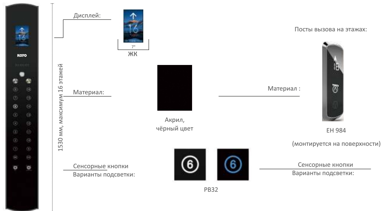
COP1070 (монтируется вровень с поверхностью)
