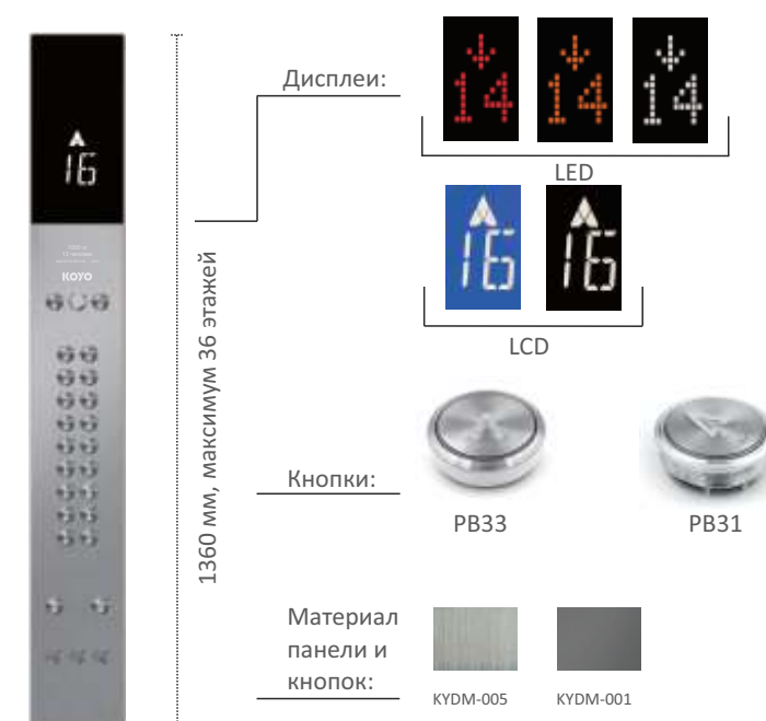
CEC260 (монтируется вровень с поверхностью)
